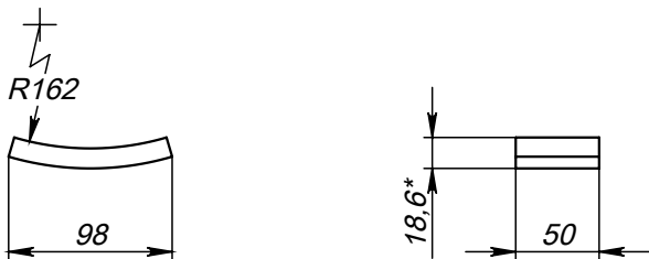
Поз2. (Упор)
